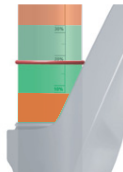
Obr. 101: Předepsaný rozsah SAG (zelený) a zakázaný rozsah SAG (červený)
