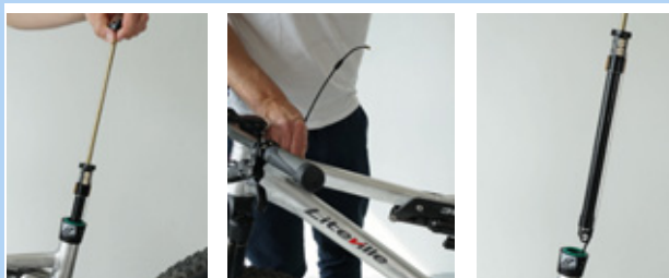
Obr. 171: Vytažení kazety
