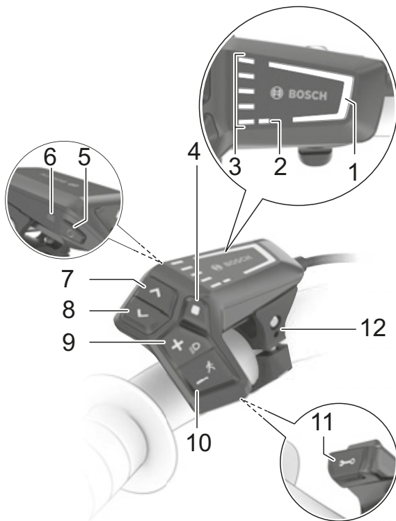
110. ábra: BOSCH LED Remote kezelőegység áttekintése
