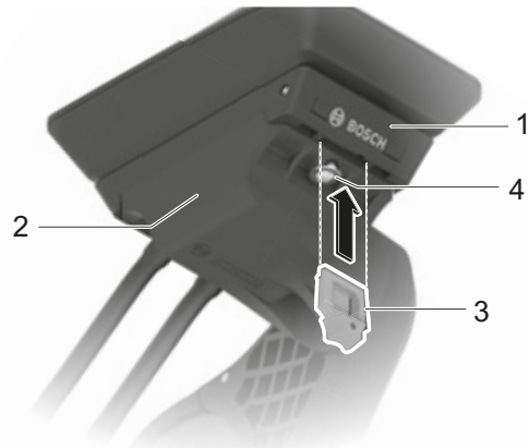
108. ábra: A vezérlőegység-csavar elhelyezkedése
