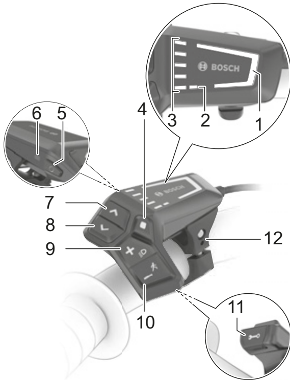
121. ábra: BOSCH LED Remote kezelőegység áttekintése
