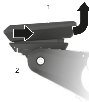
109. ábra: A fedélzeti számítógép levétele
