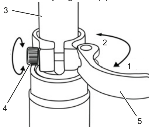
73. ábra: A nyeregcső gyorszárjának nyitása
