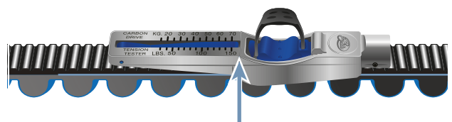
Figura 181: Calibro di verifica sulla cinghia
