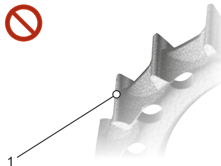
Figura 178: Profilo usurato dei denti
