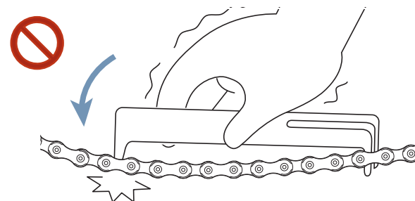
Figura 175: Il calibro di misura dell'usura entra tra due maglie
