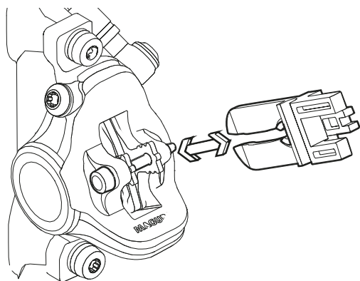
Figura 62: Fissaggio della sicura di trasporto
