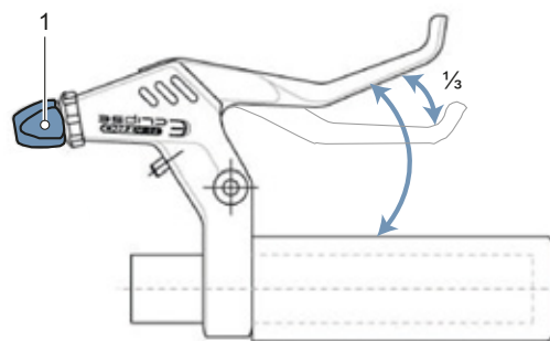
Figura 165: Ruotare la vite di regolazione (1) finché l'azione frenante non inizia in corrispondenza di \frac{1}{3} della corsa del freno a mano
