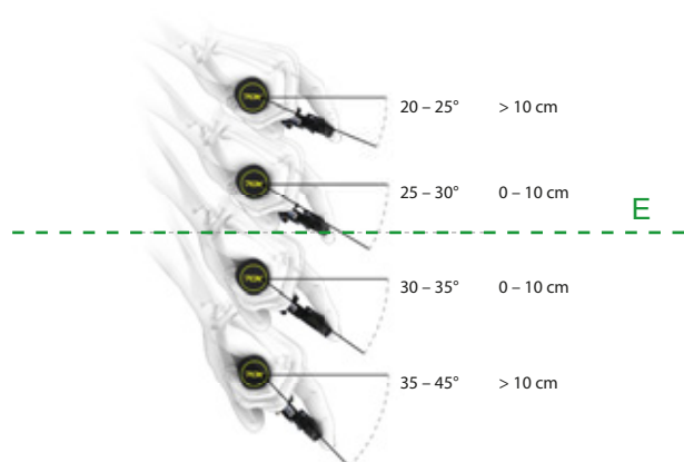
Figura 120: Angolo di inclinazione della leva del freno
