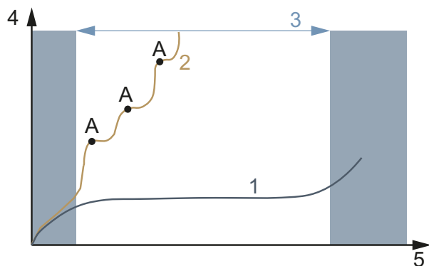
Figura 158: Diagramma dell'usura, asportazione di materiale (y) in funzione della durata di funzionamento (x)
