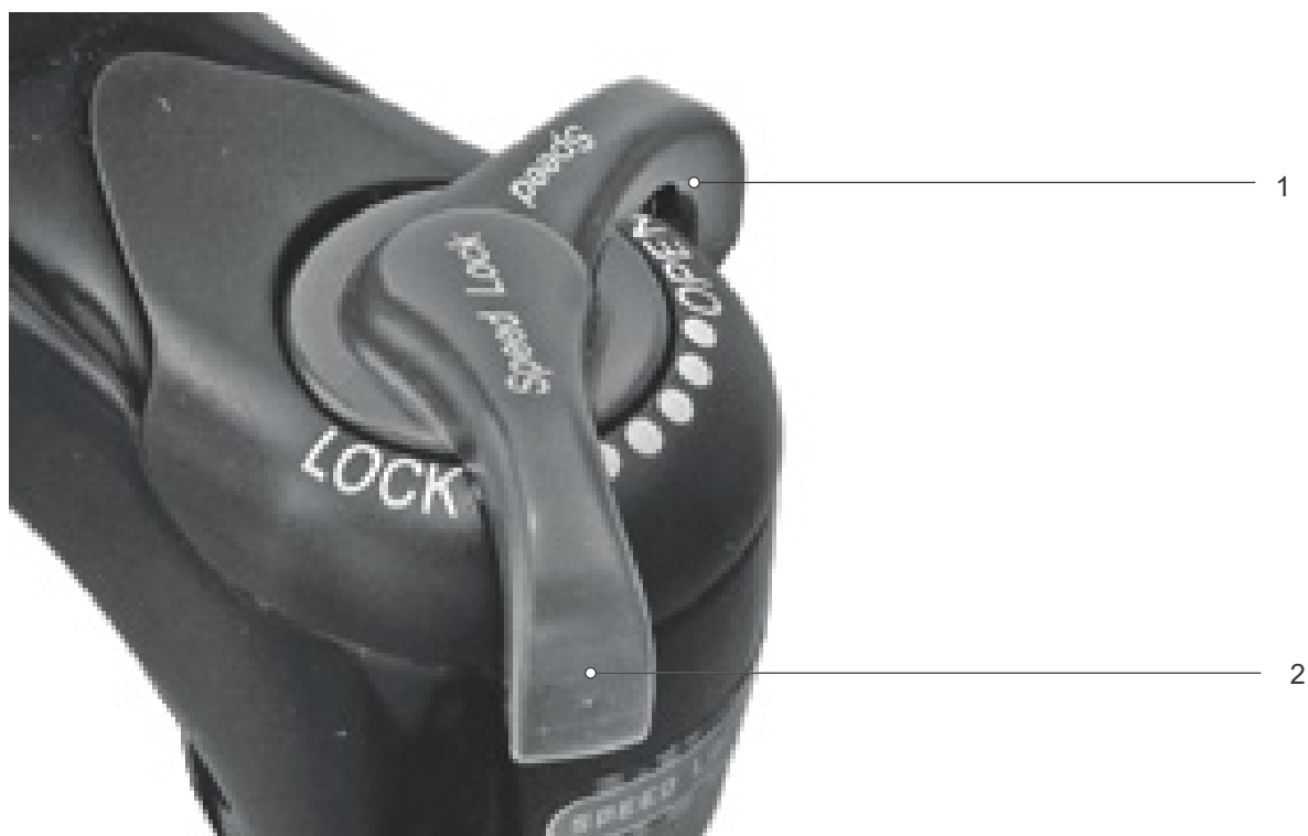
Figura 151: Ammortizzatore a stadi di pressione SR SUNTOUR in posizione aperta (1) e chiusa (2)
