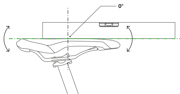
Figura 106: Sella in posizione orizzontale con angolo di inclinazione di 0° del centro della sella
