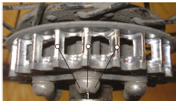
Figura 179: Esempio: profilo usurato dei denti
