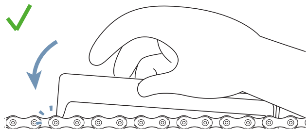
Figura 174: Il calibro di misura dell'usura non entra tra le maglie
