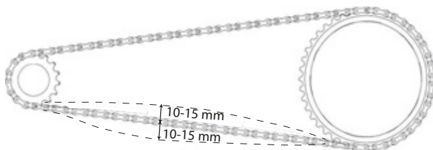
Figura 166: Controllo della tensione della catena, esempio: 5 mm verso l'alto, 10 mm verso il basso = scostamento 15 mm
