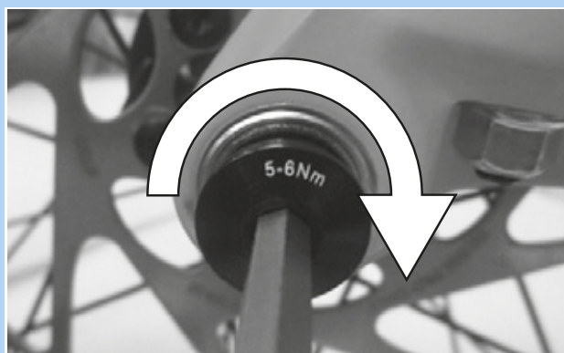
Figura 68: Serraggio della vite di sicurezza
