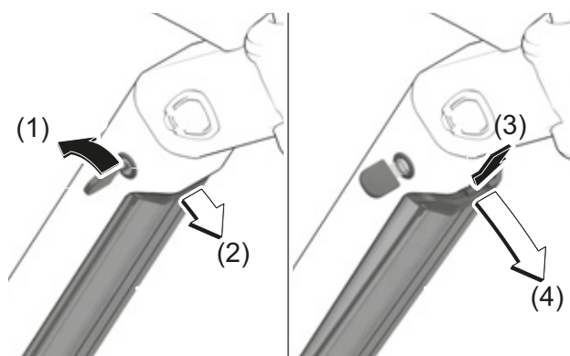
Figura 143: Smontaggio della batteria
