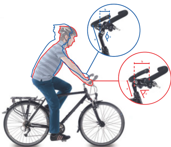
Figura 114: Posizione per bicicletta da città (blu) e per bicicletta da trekking (rosso) tramite modifica dell'angolo
