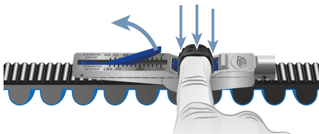
Figura 182: Spinta del calibro di verifica verso il basso con il dito
