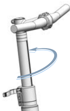
Figura 138: Esempio: All Up posizionato per la marcia
