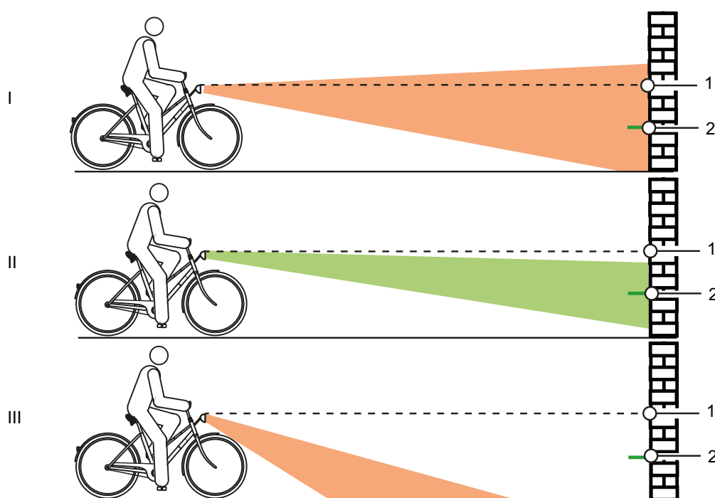
Figura 129: Luce regolata a un'altezza eccessiva (1), correttamente (2) e a un'altezza insufficiente (3)
