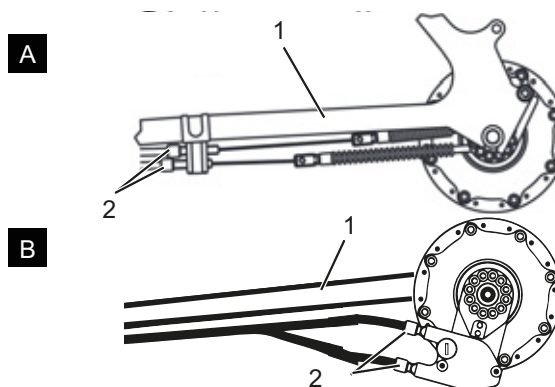
Figura 191: Boccole di regolazione (2) di due versioni alternative (A e B) di un cambio azionato da cavo doppio sul fodero orizzontale (1)
