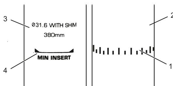
Figura 103: Particolare dei cannotti reggisella, esempi di segno indicante la minima profondità di inserimento
