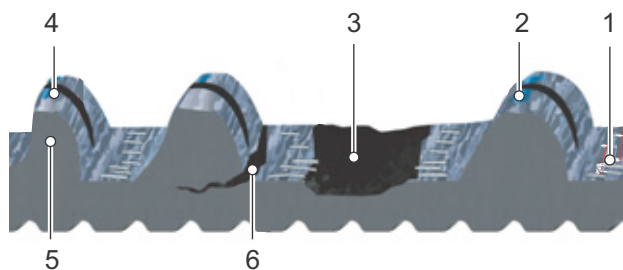
Figura 176: Caratteristiche di usura di una cinghia
