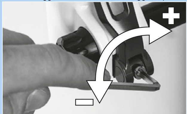
Figura 194: Regolazione della forza di serraggio del bloccaggio rapido
