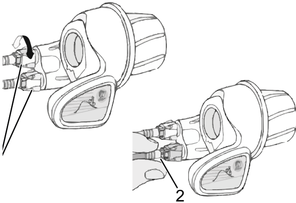
Figura 192: Interruttore a manopola del cambio con boccole di regolazione (1) e gioco della boccola del cambio (2)
