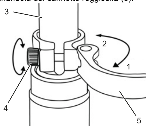
Figura 102: Apertura del bloccaggio rapido del canotto reggisella
