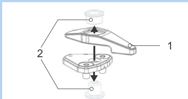
Figura 82: Collegamento della leva di sicurezza alla piastra di base
